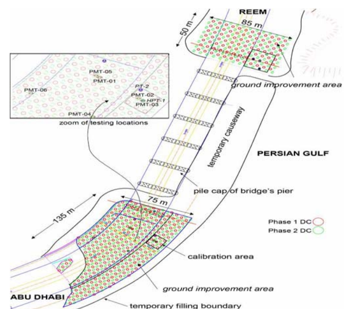
Fig. 1. Site Plan.
